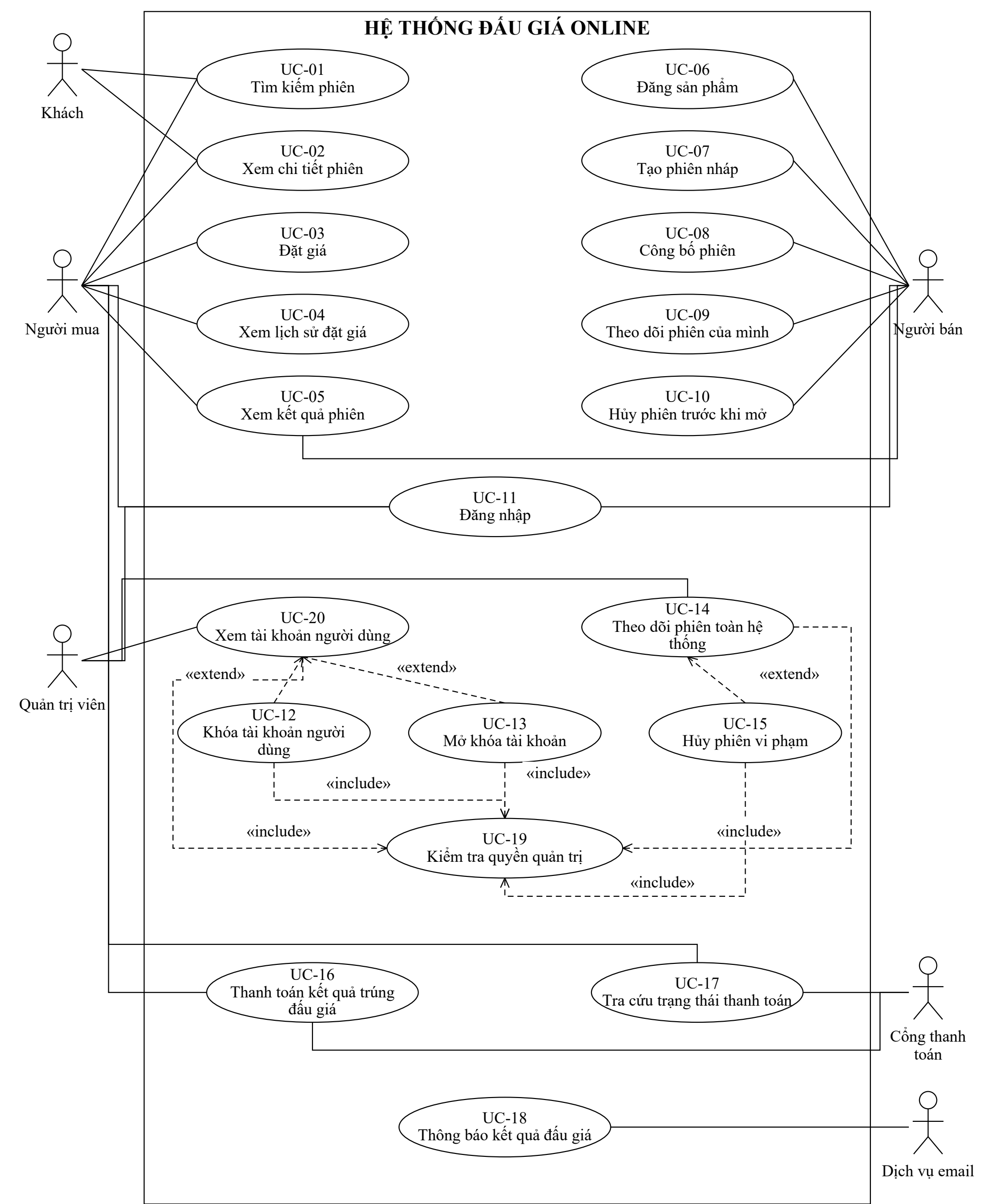
Hình 1. Sơ đồ Use Case hệ thống đấu giá online
